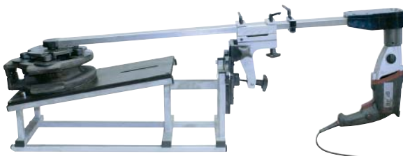
SLIM 300 beim Schleifen eines Schieberkeils
